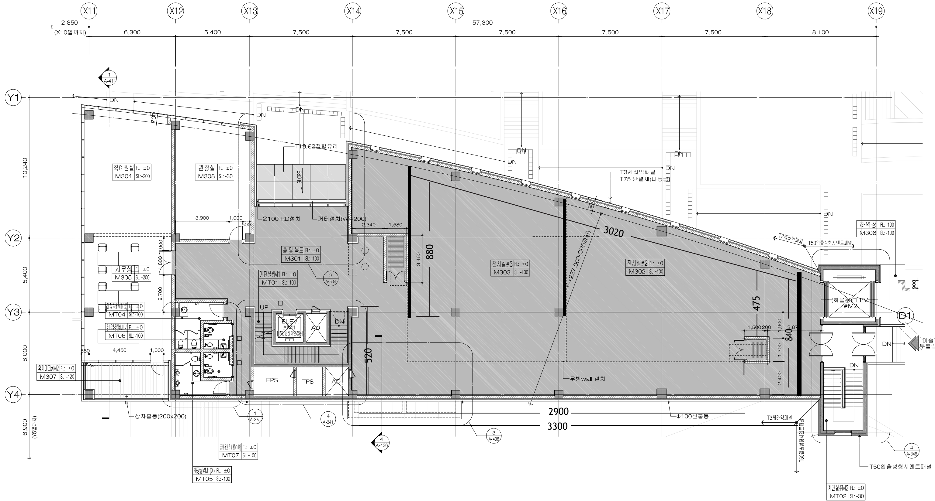
1 지상 3층 확대평면도-4 s=1/100
