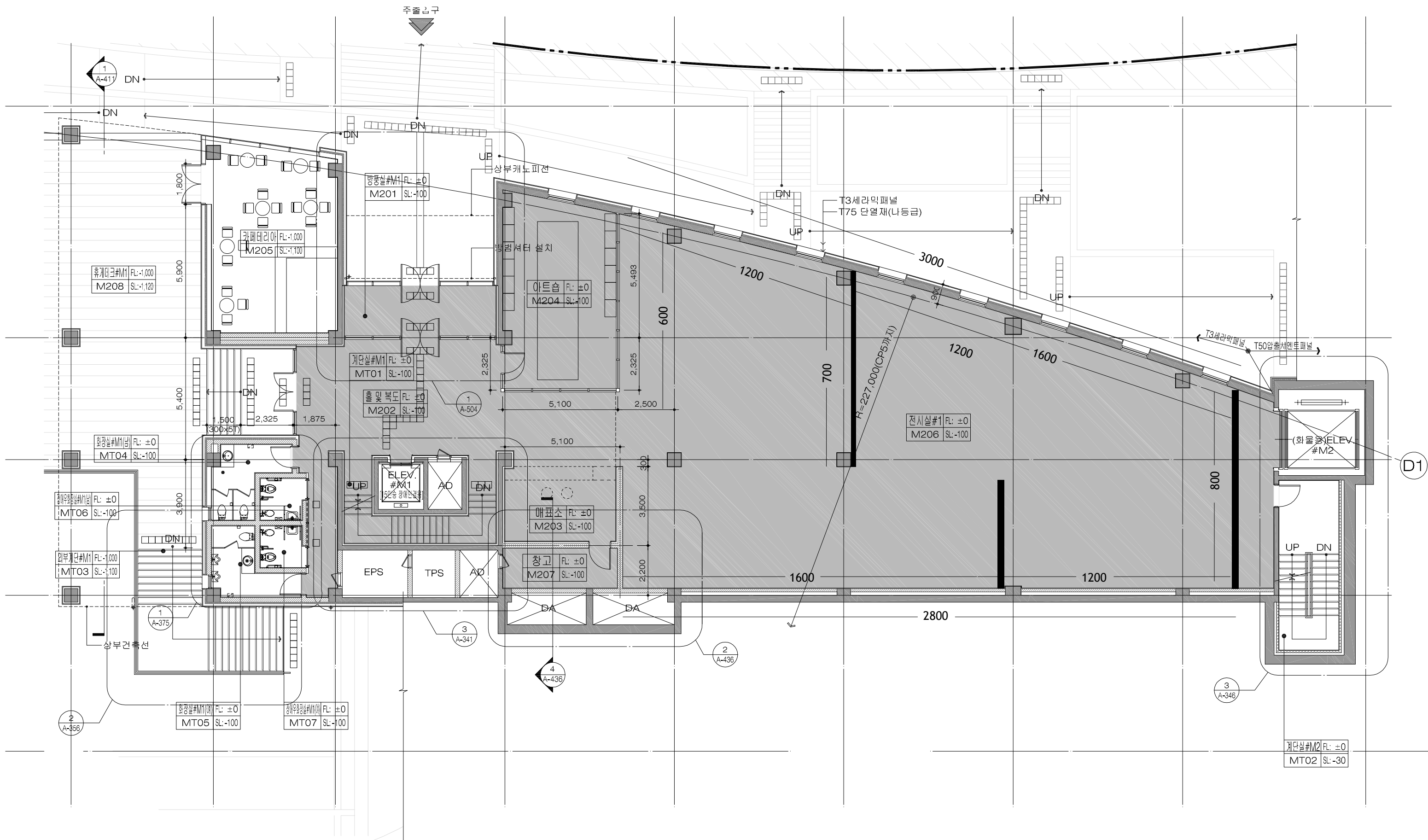
1 지상 2층 확대평면도-4 s=1/100
